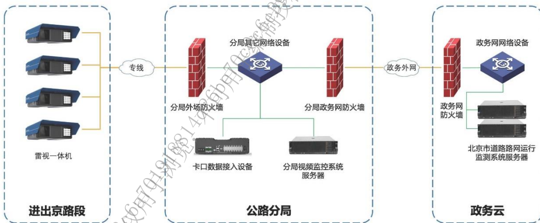
图 4.1 数据传输网络拓扑图
